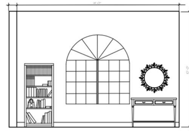
BEDROOM/ ELEVATION B SCALE: 1/8" = 1'-0"
