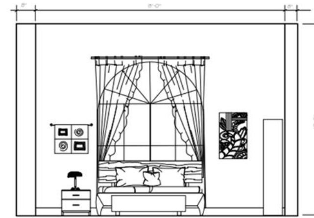
BEDROOM/ ELEVATION A SCALE: 1/8" = 1'-0"
